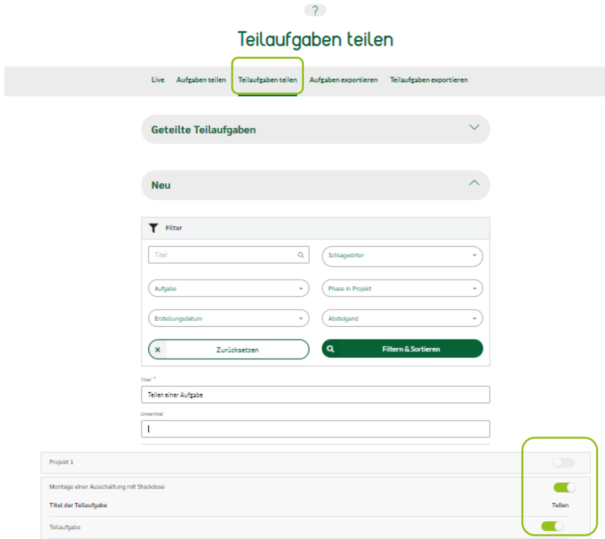
Abb. 2: Auswahlmaske – die Auswahl der Teilaufgaben erfolgt über die Schieberegler
